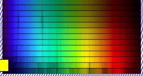
Spektrum einer Galaxie
