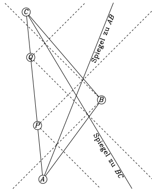
Abbildung 15: Das Zwillingsparadoxon
