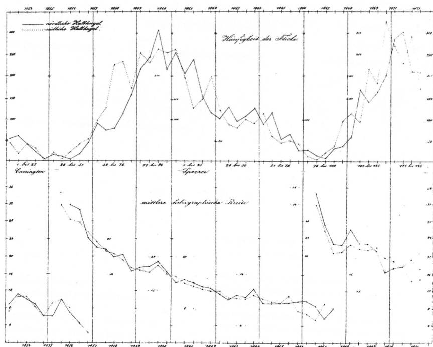
Bild 12. Ankamer Sonnenfleckenstatistik mit Häufigkeit (oben) und gemittelter heliographischer Breite (unten) der Sonnenflecken für 1854 – 1871. Nord- und Südhemisphäre der Sonne jeweils getrennt. Quelle: Spörer (1874).
