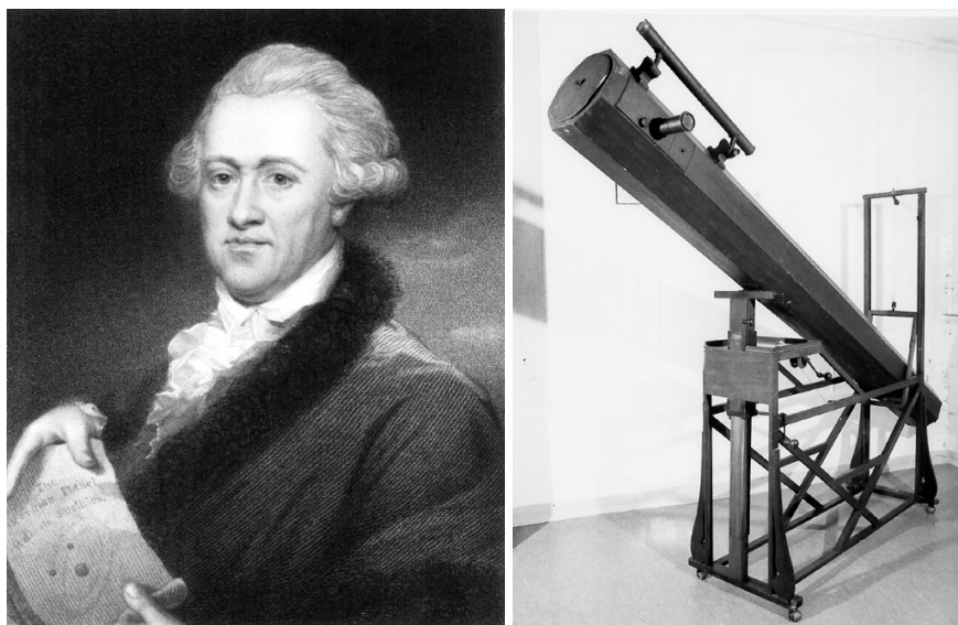
Bild 1. Friedrich Wilhelm Herschel (1738–1822); 10-füßiges Teleskop von Herschel (22-cm-Metallspiegel, rechts); mit solch einem Instrument wurden die 1801 veröffentlichten Sonnenfleckbeobachtungen unternommen. Insgesamt beobachtete Herschel fast 40 Jahre die „openings“ in der Sonnenoberfläche. 3 Photo: Universitäts-Sternwarte Göttingen.
